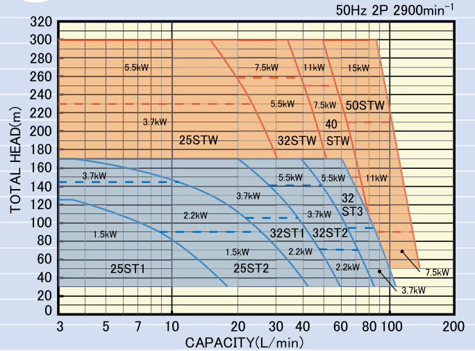
予想曲線 / Pump Supposition Curve.
